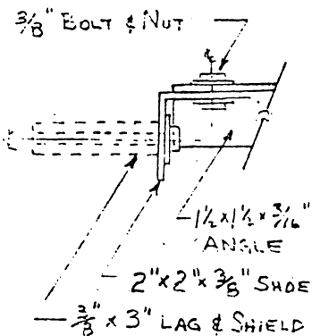
DETAIL "A" TYP (2) SCALE: 1/4" = 1"
