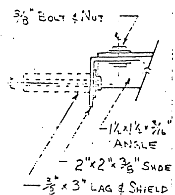
DETAIL "A" TYP (2) SCALE: 1/4" = 1"
